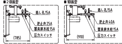
※4: 水道直結型の接続と寸法
