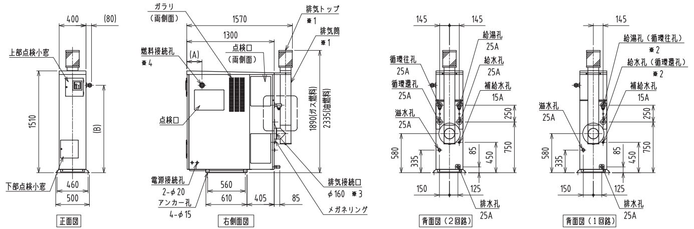
※4: 燃料接続孔位置と寸法
