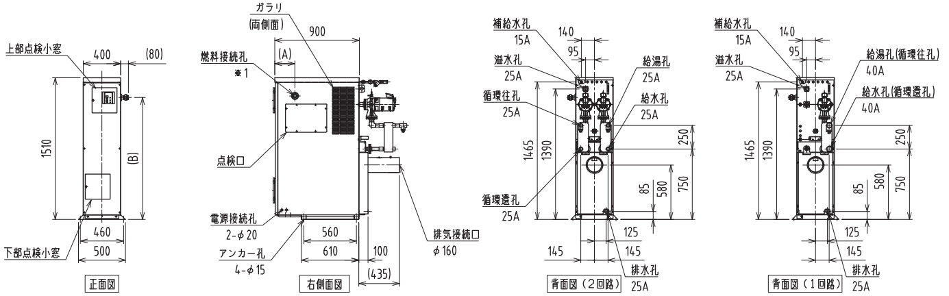
※1: 燃料接続孔位置と寸法
