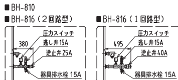
※6: 水道直結型の接続と寸法
