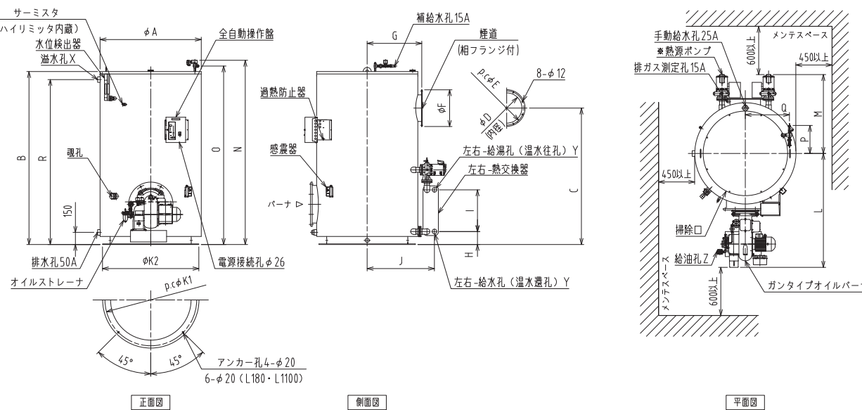
BH-L148～1100(屋内型)
