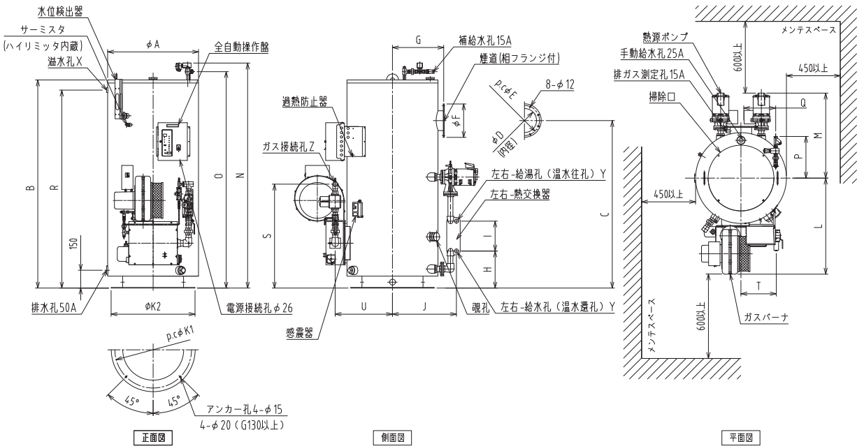
BH-G148～1100(屋内型)
