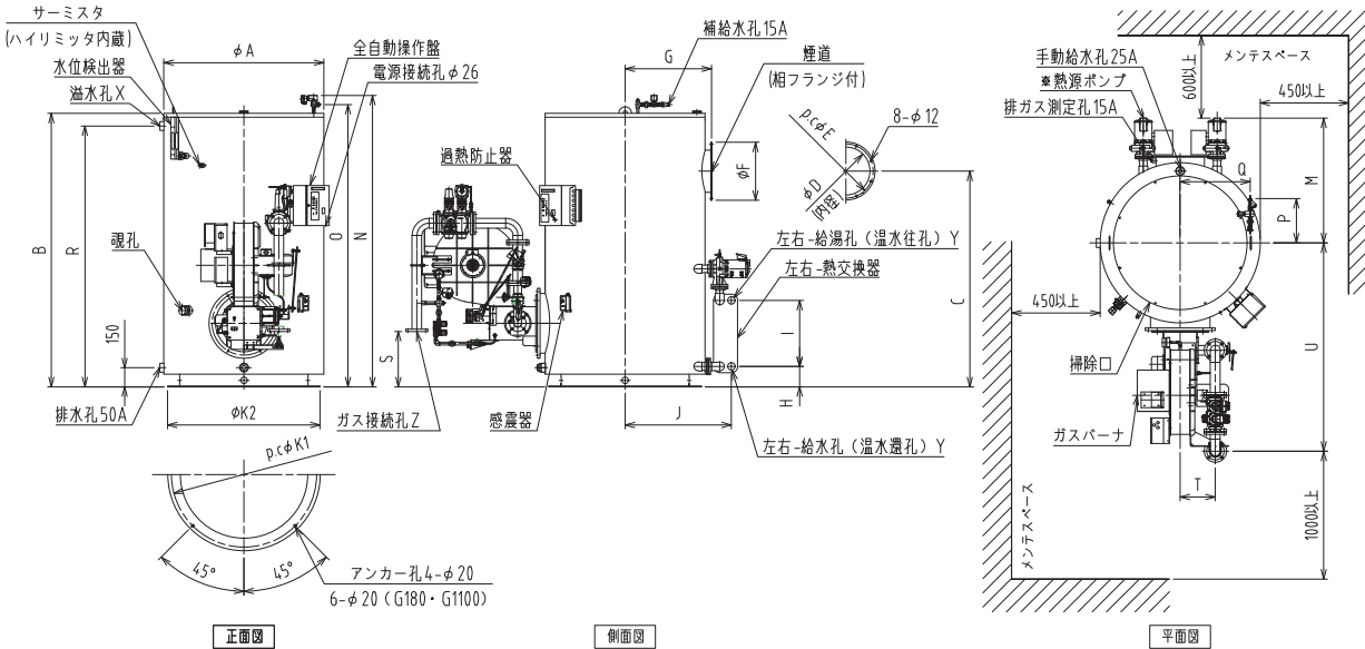
BH-G148～1100(屋内型)
