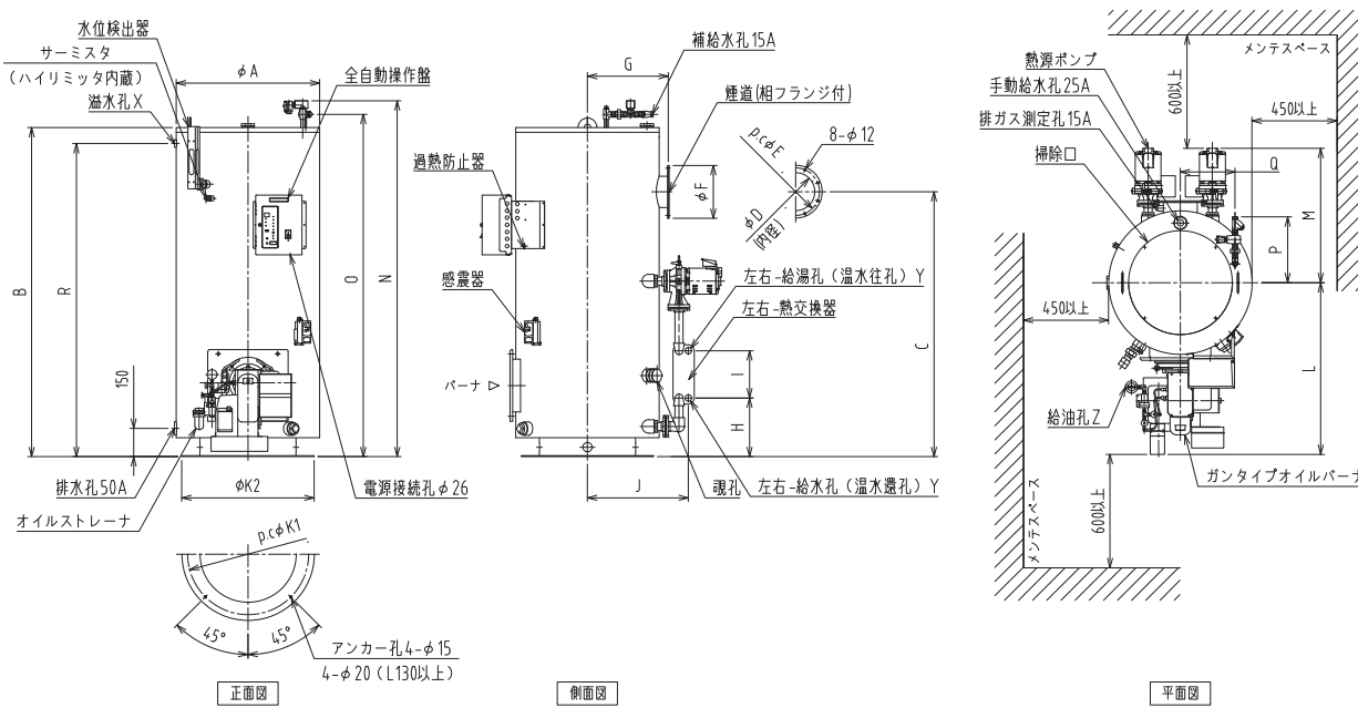
BH-L148～1100(屋内型)
