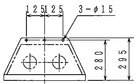
吊りブラケット取付寸法
